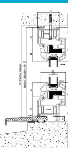
Pièce d'appui de 100 mm en base (possible en 70 et 123 mm)
