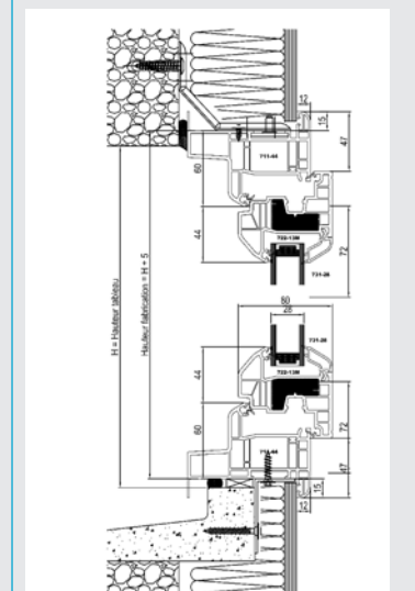
Isolation intérieure de 100 mm (possible de 70 à 180 mm)
