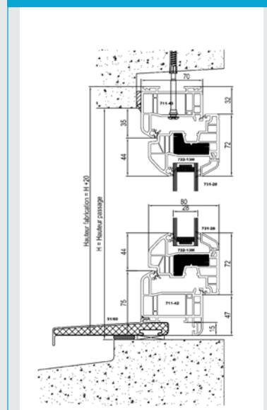
Dormant de 70 mm et pièce d'appui rapportée dépassant de 100 mm
