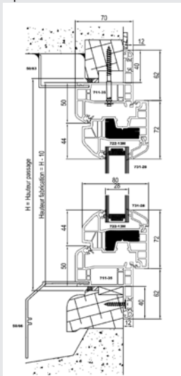
Ailette rénovation de 40 mm en base (possible en aile de 27 et 60 mm)
